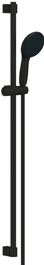
261632433 | N/A Tempesta 110 • 900 mm duschstång • 110 mm duschhuvud • 2 stråltypen (Rain, Jet) • Flöde (3 bar) 8,5 l/min
