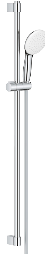
27925003 | 8233332 Tempesta 110 • 900 mm duschstång • 110 mm duschhuvud • 1 stråltyp (Rain) • Flöde (3 bar) 7,6 l/min
