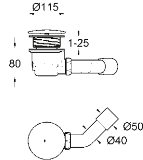
49 534 000* Universallås för universella duschkar
