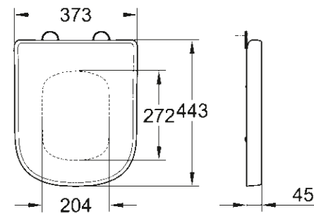
39 330 000 Sits & Lock mjukstänging Snabbkoppling 39 331 000 utan mjukstängning
