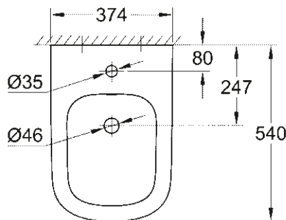
39 208 000 39 208 00H* Vägghängd bidé
