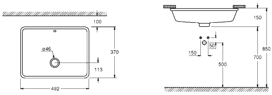
39 480 00H Underlimmat tvättställ 50 cm
