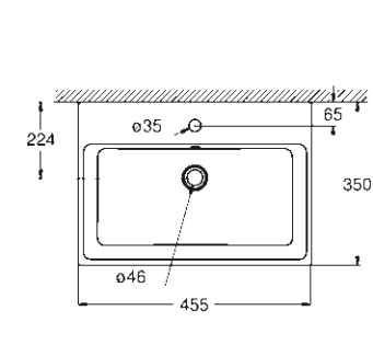
39 483 00H Handskölj möbeltvättställ 45 cm
