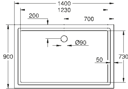
39 307 000* Universellt duschkar 90 cm x 140 cm
