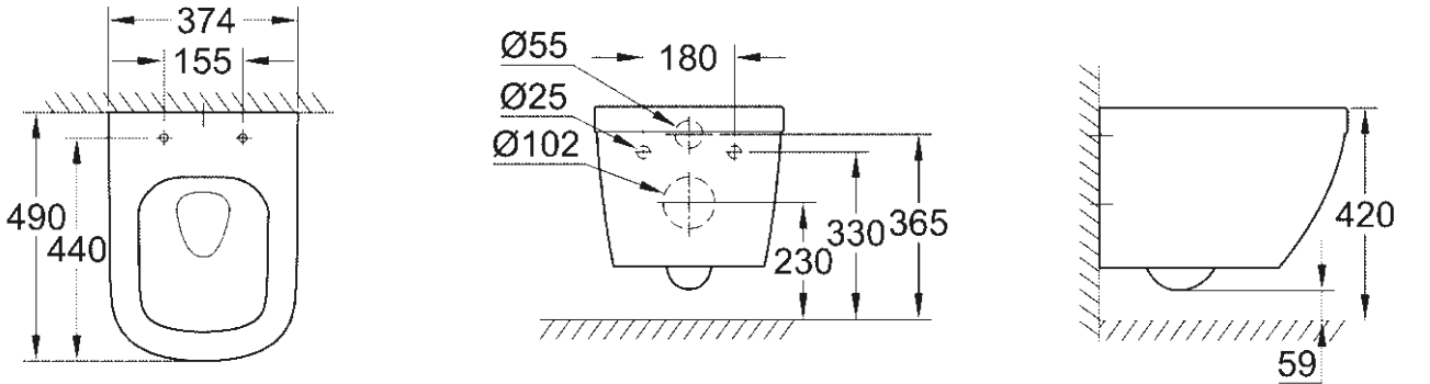
39 206 000 39 206 00H* Kompakt vägghängd toalett Triple Vortex spolning
