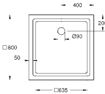
39 302 000* Universellt duschkar 80 cm x 80 cm
