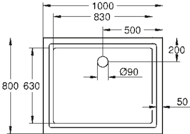
39 306 000* Universellt duschkar 80 cm x 100 cm
