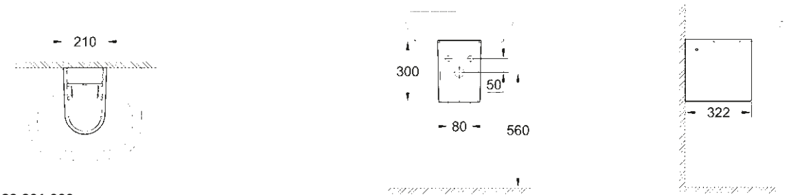
39 201 000 Halvfristående piedestal för tvättställ
