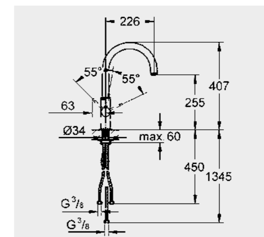
Waga armatury
