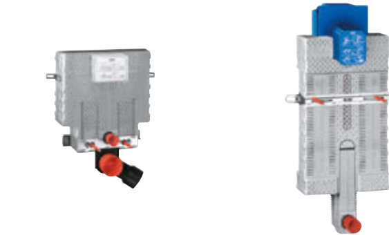
38 415 001 Uniset for toalett med sisterner 6 – 9 l dobbelspyling / start og stopp / enkelspyling, vanntilførsel fra venstre, høyre eller toppen, aktivering i front eller på toppen 0,82 m installasjonshøyde
