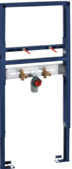
39 052 000 Rapid SL for servant høyden kan justeres, for etthullsinstallasjon, 1,13 m installasjonshøyde for installasjon på veggen eller stendervegg, to støydpende tilkoblinger 1/2"
