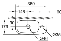
39 324 000 39 324 00H* Fontein 45 cm
