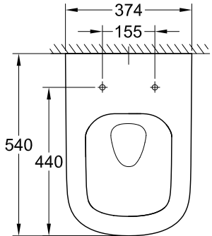
39 328 000 39 328 00H* Hangende WC
