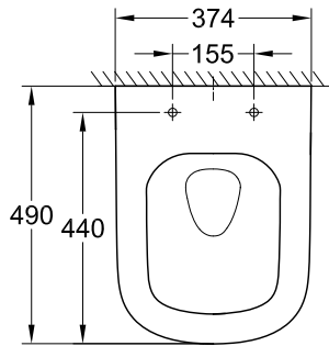
39 206 000 39 206 00H* Compacte hangende WC
