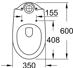
39 428 000 Staande WC, naadloos gekoppeld, horizontale afvoer
