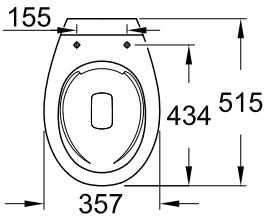
39 431 000 Staande WC, verticale afvoer
