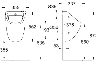
39 438 000 Urinoir met verborgen toevoer
