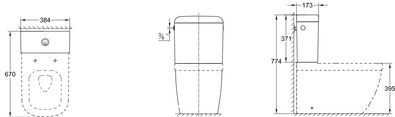
39 333 000 Spoelreservoir met toevoer en afvoer aan de zij- en achterkant
