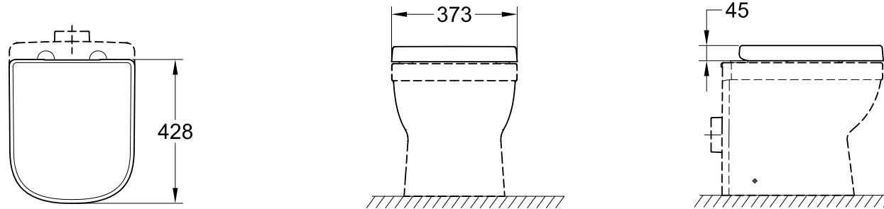
39 458 000 Softclose zitting en deksel voor compact toilet
