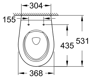
39 427 000 Hangende WC, horizontale afvoer
