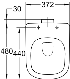
39 329 000 39 329 00H* Staande WC, universele afvoer
