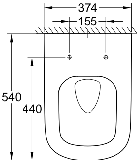
39 339 000 39 339 00H* Staande WC, achterkant tegen de muur, universele afvoer
