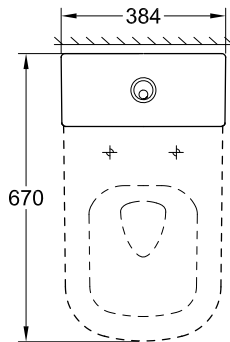
39 332 000 Spoelreservoir met toevoer van onderaf
