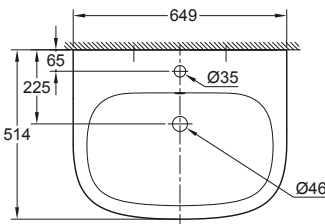
39 323 000 39 323 00H* Hangende wastafel 65 cm
