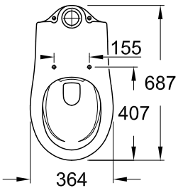
39 429 000 Staande WC, naadloos gekoppeld, verticale afvoer
