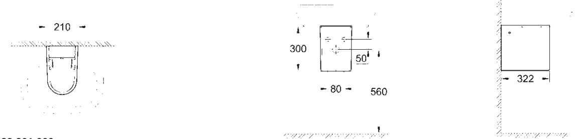
39 201 000 Halve zuil voor wastafels
