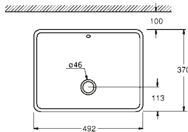
39 480 00H Onderbouwwastafel 50 cm
