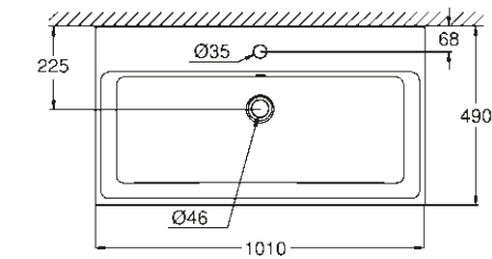
39 386 00H Hangende wastafel 100 cm
