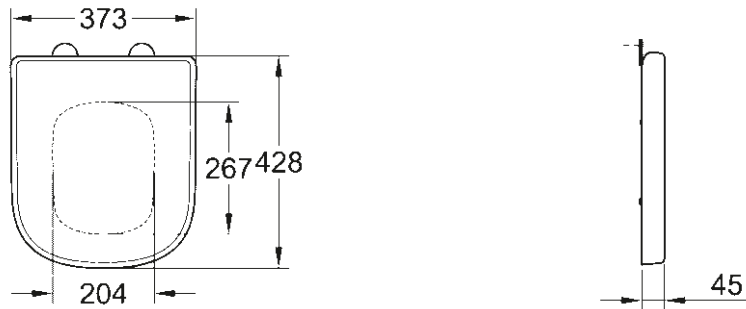
39 458 000 Softclose zitting en deksel voor compact toilet Gemakkelijk te verwijderen zitting 39 459 000 Zonder Softclose
