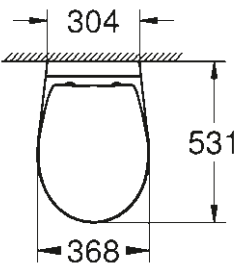
39 351 000 Hangtoilet randloos Softclose zitting en deksel Gemakkelijk te verwijderen zitting
