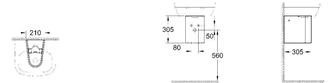
39 325 000 Sifonkap voor fontein 45 cm
