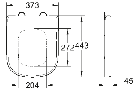
39 330 000 Softclose zitting en deksel Gemakkelijk te verwijderen zitting 39 331 000 Zonder Softclose
