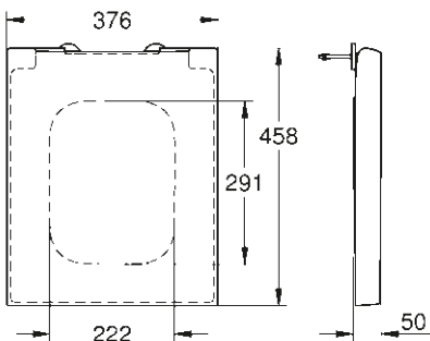
39 488 000 Softclose zitting en deksel Gemakkelijk te verwijderen zitting
