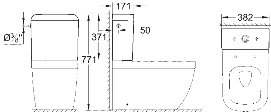
39 333 000 Spoelreservoir met toevoer aan de zij- en achterkant
