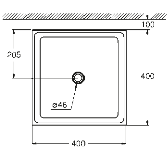
39 482 00H Vrijstaande opbouw wastafel 40 cm
