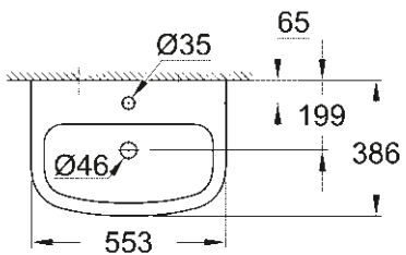
39 440 000 Hangende wastafel 55 cm
