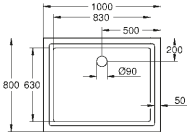
39 306 000* Universele douchevloer 80 x 100 cm
