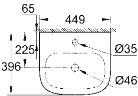
39 324 000 39 324 00H* Fontein 45 cm
