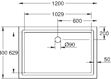
39 305 000* Universele douchevloer 80 x 120 cm
