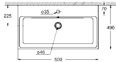
39 478 00H Opbouwwastafel 50 cm
