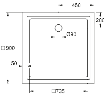
39 301 000* Universele douchevloer 90 x 90 cm
