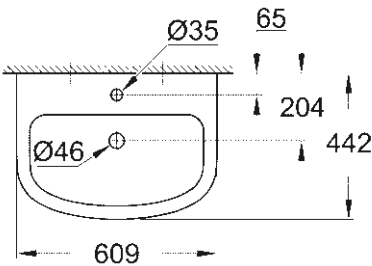
39 420 000 Hangende wastafel 65 cm
