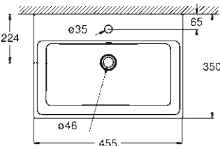
39 483 00H Fontein 45 cm
