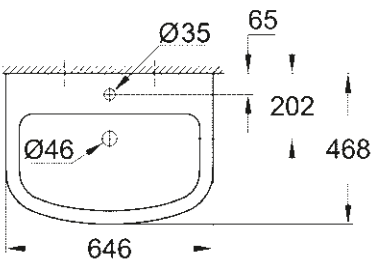
39 420 000 Hangende wastafel 65 cm
