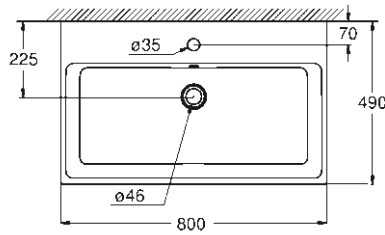
39 469 00H Hangende wastafel 80 cm
