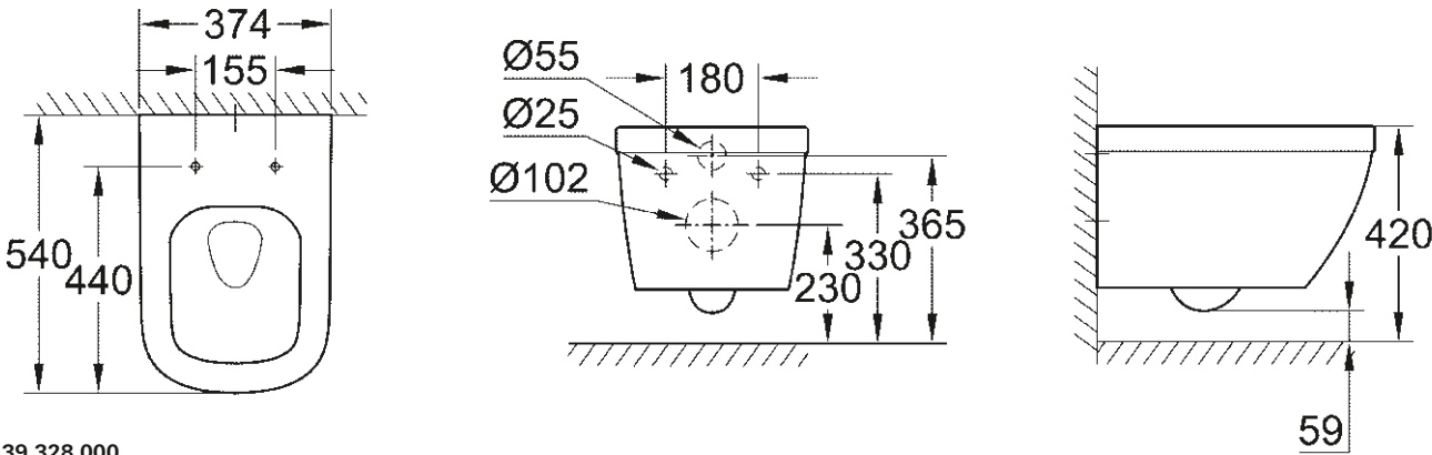
39 328 000 39 328 00H* Hangtoilet Triple Vortex
