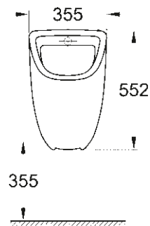
39 438 000 Urinoir met verborgen toevoer
