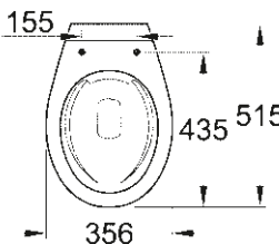
39 430 000 Staand toilet randloos
