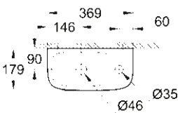
39 327 000 39 327 00H* Mini-handwastafel 37 cm
