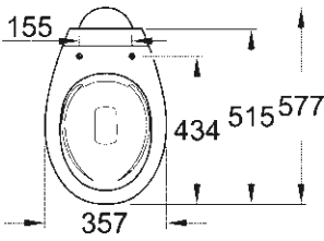
39 431 000 Staand toilet randloos
