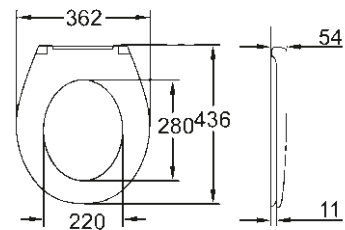
39 493 000 Softclose zitting en deksel Gemakkelijk te verwijderen zitting 39 492 000 Zonder Softclose Gemakkelijk te verwijderen zitting
