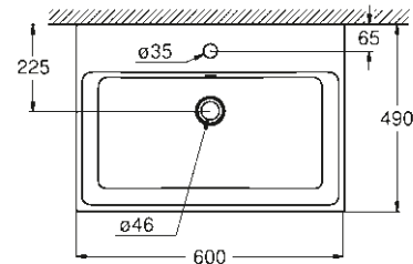
39 473 00H Hangende wastafel 60 cm
