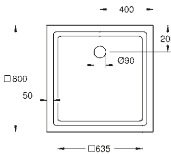
39 302 000* Universele douchevloer 80 x 80 cm
