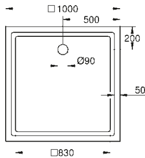
39 300 000* Universele douchevloer 100 x 100 cm
