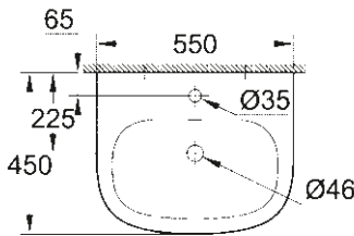
39 336 000 39 336 00H* Hangende wastafel 55 cm
