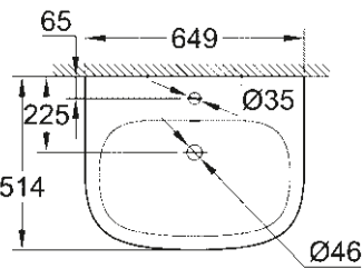
39 323 000 39 323 00H* Hangende wastafel 65 cm
