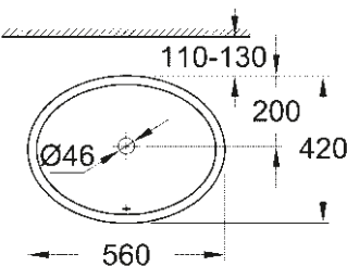
39 423 000 Onderbouw wastafel 55 cm
