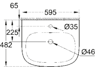
39 335 000 39 335 00H* Hangende wastafel 60 cm
