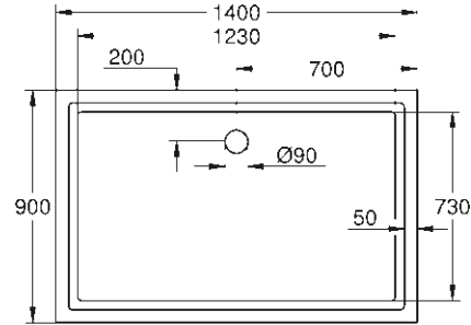
39 307 000* Universele douchevloer 90 x 140 cm
