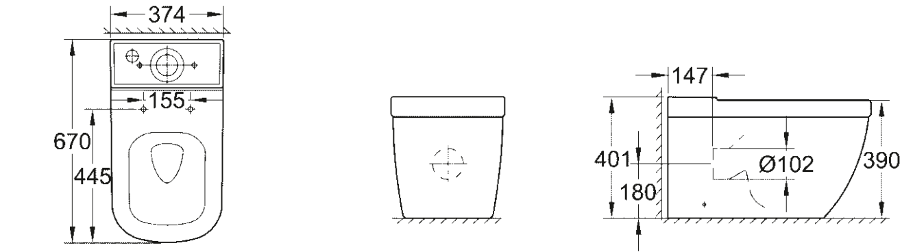
39 338 000 39 338 00H* Staand toilet voor naadloos gekoppelde combinatie Triple Vortex, universele afvoer
