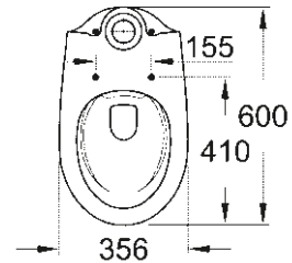
39 349 000 Staand toilet voor naadloos gekoppelde combinatie randloos, horizontale afvoer
