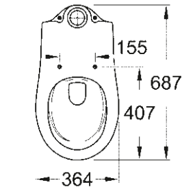
39 429 000 Staand toilet voor naadloos gekoppelde combinatie randloos, verticale afvoer
