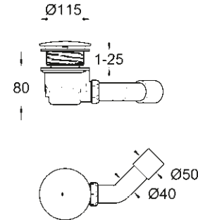
49 534 000* Afvoergarnituur horizontaal voor universele douchevloeren
