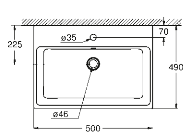
39 474 00H Hangende wastafel 50 cm
