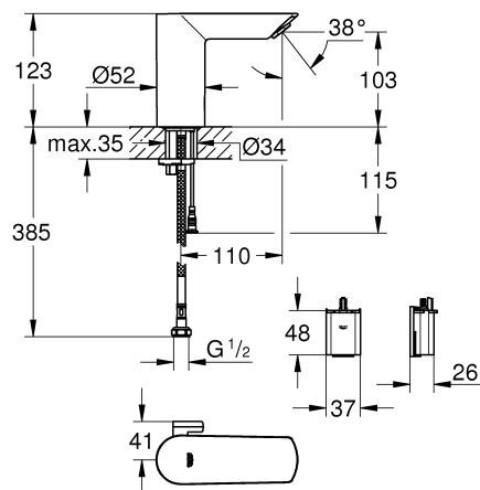
BAU COSMOPOLITAN E 36451000
