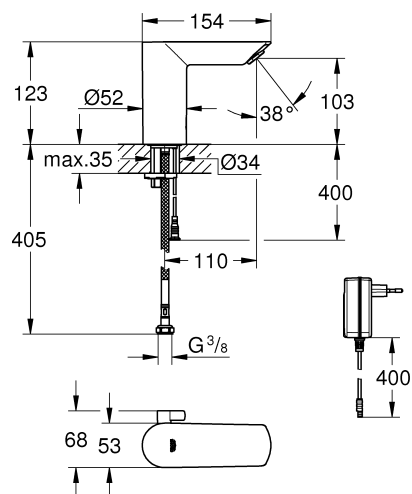
BAU COSMOPOLITAN E 36453000
