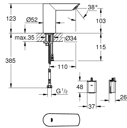
BAU COSMOPOLITAN E 36452000
