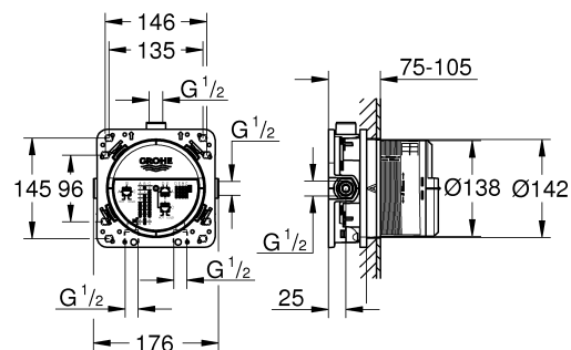
GROHE RAPIDO SMARTBOX 35600000
