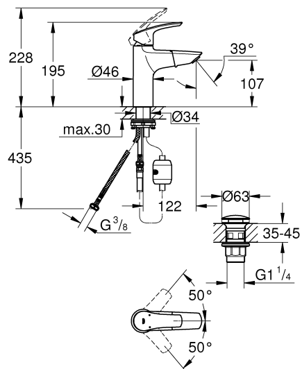
BAU COSMOPOLITAN E 36451000
