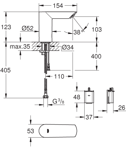
BAU COSMOPOLITAN E 36452000
