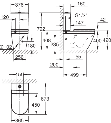
EURO CERAMIC 102513SH00
