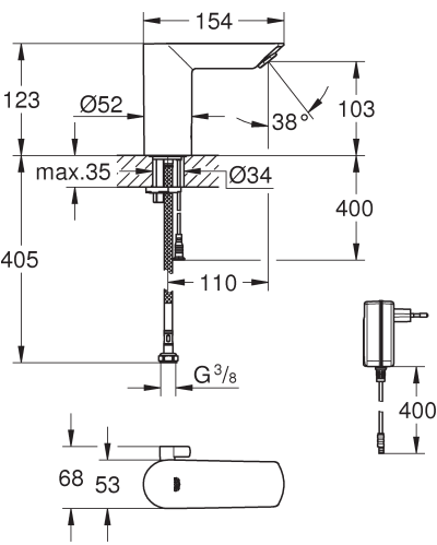
BAU COSMOPOLITAN E 36453000
