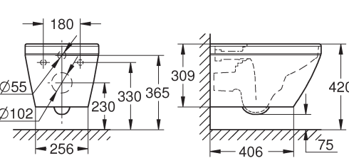
EURO CERAMIC 102485SH00
