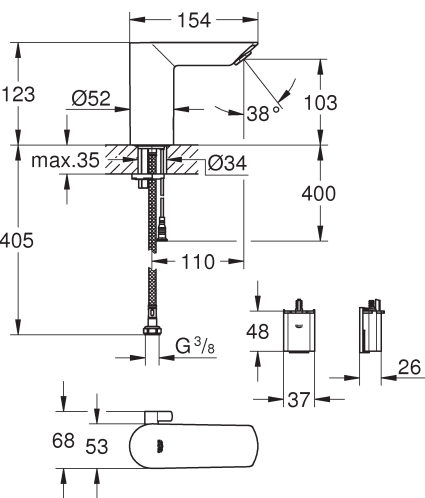
BAU COSMOPOLITAN E 36451000
