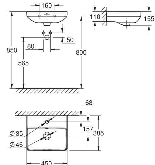
EURO CERAMIC 102435SH00
