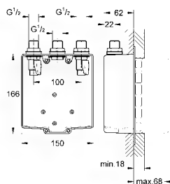
36 322 000 Subconjunto para empotrar para ref. 36 321 000.
