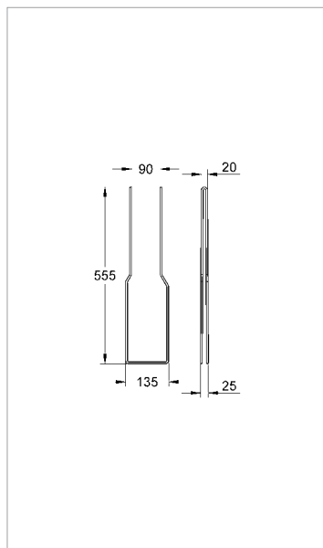
37 573 000 Uniset soportes para WC y Bidé, autoportantes.
