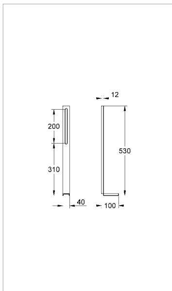
37 304 000 Uniset pies de apoyo para WC y Bidé. Instalación delante de pared resistente.
