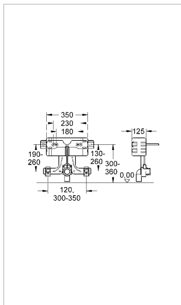
37 578 001 Uniset para bidé.
