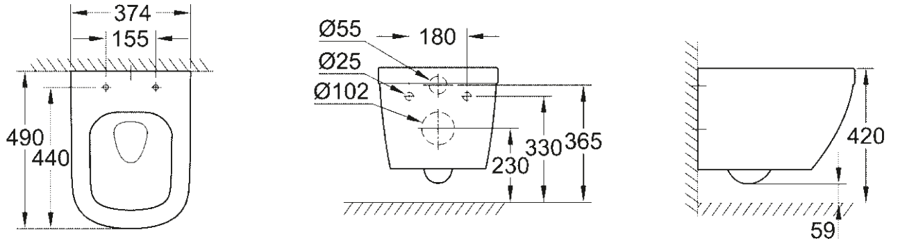
39 206 000 39 206 00H* Compact wall hung WC rimless
