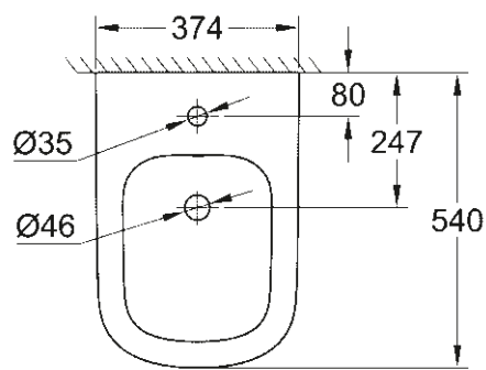
39 340 000 39 340 00H* Floorstanding bidet
