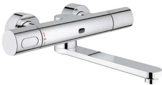
36 332 000 | 704163204 Eurosmart Cosmopolitan E | 297 mm fremspring | 6V batteri | Infrarød sensor | Vægmonteret | Med termostat | GROHE CoolTouch skoldningsikker | 8,0 l/min
