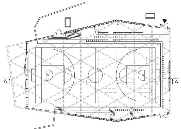
Grundriss Erdgeschoss, M 1:500
