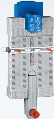
38 785 000 Uniset Element für Urinal mit Infrarot-Elektronik
