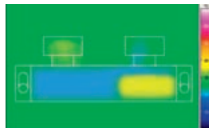
Image thermique avec GROHE CoolTouch®
