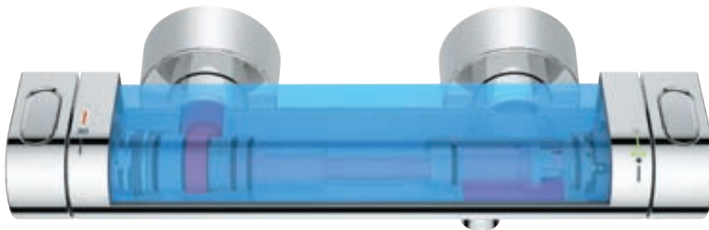
Boîtier de sécurité avec canal de refroidissement
