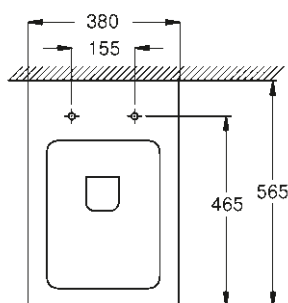
39 485 00H Vas de WC cu montare pe podea lipit de perete, rimless
