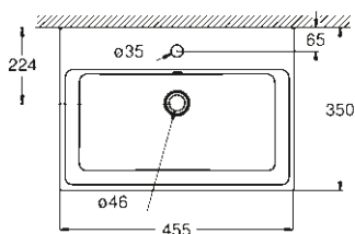
39 483 00H Lavoar de serviciu 45 cm
