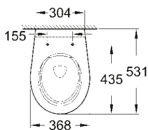
39 427 000 Wall hung WC rimless
