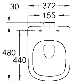
39 329 000 39 329 00H* Floorstanding WC rimless
