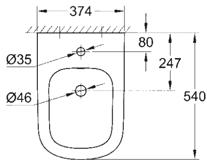
39 208 000 39 208 00H* Wall hung bidet
