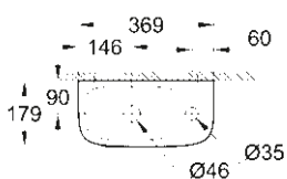
39 327 000 39 327 00H* Mini handrinse basin 37 cm
