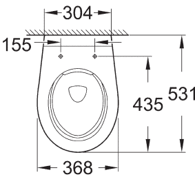
39 427 000 Wall hung WC rimless
