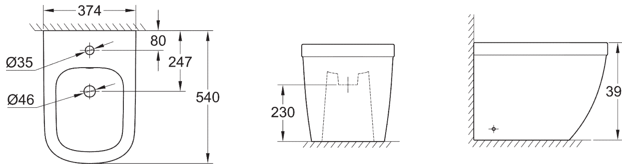
39 340 000 39 340 00H* Floorstanding bidet
