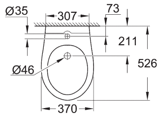
39 433 000 Wall hung bidet
