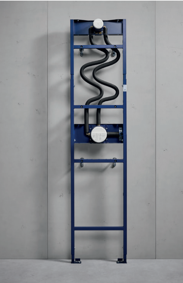
GROHE RAPIDO SHOWER FRAME
