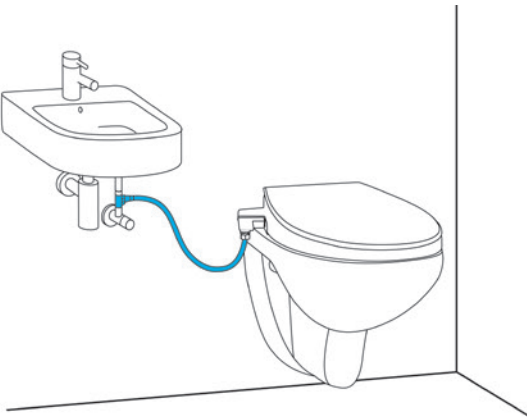
AANSLUITING OP DE WATERTOEOVOER VAN EEN WASTAFEL
