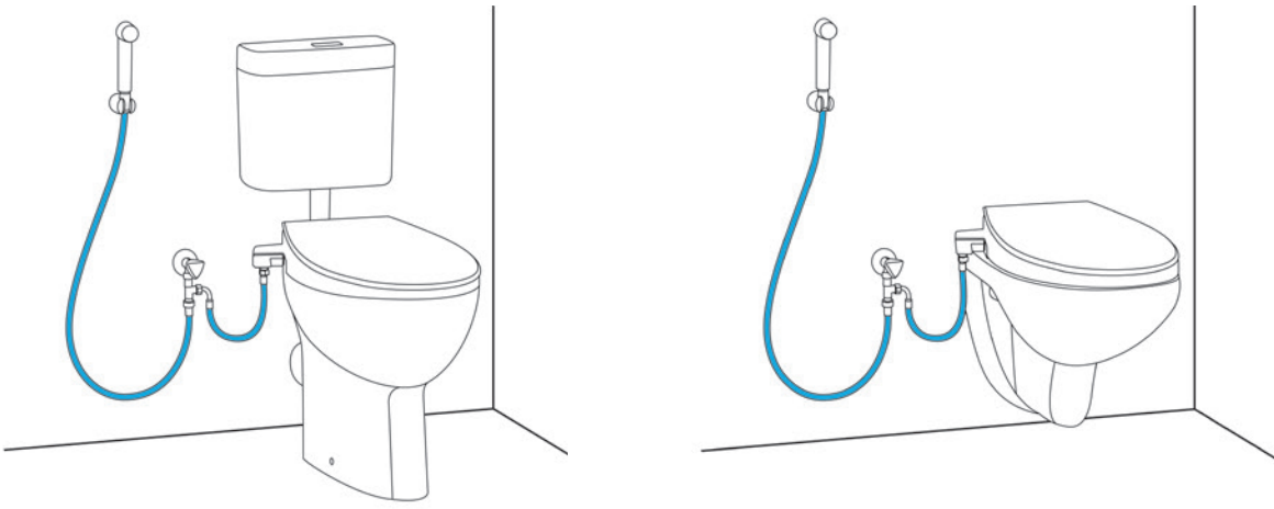
AANSLUITING OP DE WATERTOEOVOER VAN EEN TRIGGER SPRAY
