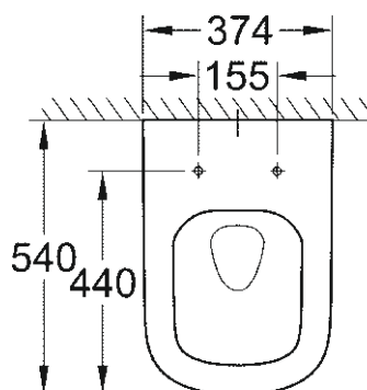
39 328 000 / 613344.000 39 328 00H * / 613344.060 Væghængt WC Triple Vortex
