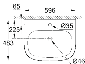
39 337 000 / 634121.000 39 337 00H* / 634121.060 Håndvask til bordtop 60 cm
