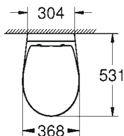
39 351 000 / 613341.200 Væghængt WC Kantløs Sæde og låg med soft close Quick release funktion
