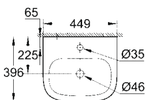
39 324 000 / 623223.000 39 324 00H* / 623223.060 Håndvaskfad 45 cm
