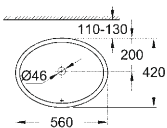
39 423 000 / 636016.600 Håndvask til bordplade, underbygget 55 cm
