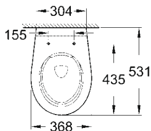
39 427 000 / 613341.000 Væghængt WC
