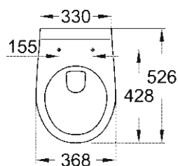
39 491 000 / 613340.000 Væghængt WC Åben kant
