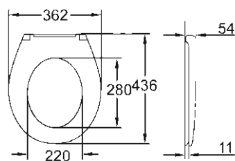
39 493 000 / 614780.100 Sæde og låg med soft close Quick release funktion 39 492 000 / 614780.200 Uden soft close Quick release funktion
