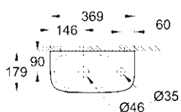
39 327 000 / 623222.200 39 327 00H* / 623222.260 Lille håndvaskfad 37 cm
