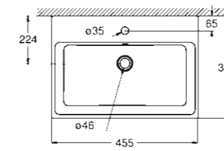
39 483 00H Lave-mains 45 cm
