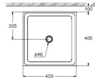
39 482 00H Vasque à poser sans trop plein 40 cm
