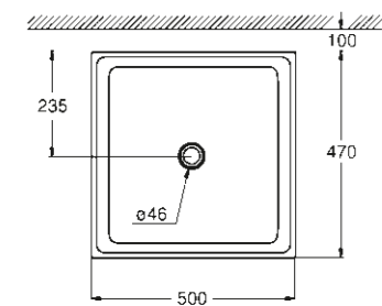
39 481 00H Vasque à poser sans trop plein 50 cm
