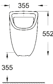
39 439 000 Urinoir avec alimentation par le dessus
