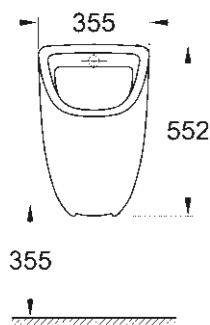
39 438 000 Urinoir avec alimentation encastrée
