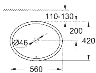
39 423 000 Vasque à encastrer par le dessous 55 cm
