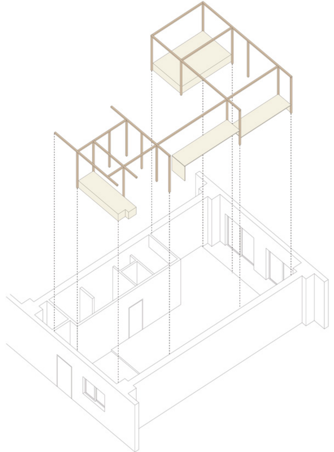
Diese Skizze des Frame House zeigt, wie die Holzbalken in die vorhandene Struktur eingefügt wurden.
