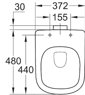
39 329 000 39 329 00H* Stand-Tiefspül-WC randlos Abgang universal
