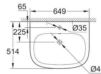
39 323 000 39 323 00H* Waschtisch 65 cm
