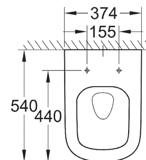
39 328 000 39 328 00H* Wand-Tiefspül-WC Triple Vortex Spülung randlos
