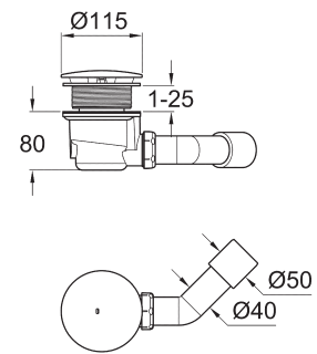
49 534 000* Duschwannenablauf, Abgang waagrecht
