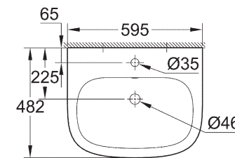
39 335 000 39 335 00H* Waschtisch 60 cm
