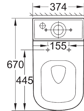
39 338 000 Stand-WC-Kombination Triple Vortex Spülung, randlos, Abgang universal
