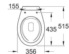
39 430 000 Stand-WC randlos Abgang waagrecht
