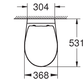
39 351 000 Set Wand-Tiefspül-WC randlos WC-Sitz mit Deckel Soft Close Quick Release Funktion – werkzeuglos abnehmbar
