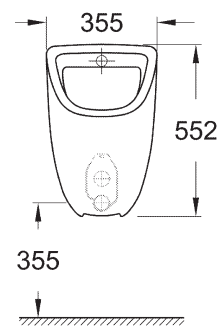
39 438 000 Urinal Zulauf verdeckt
