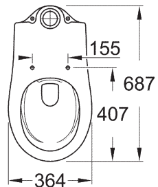
39 429 000 Stand-WC-Kombination randlos Abgang senkrecht
