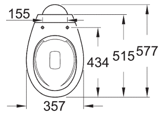
39 431 000 Stand-WC randlos Abgang senkrecht
