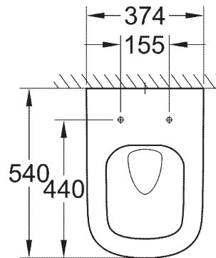
39 339 000 39 339 00H* Stand-Tiefspül-WC back to wall Triple Vortex Spülung randlos
