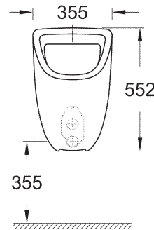
39 439 000 Urinal Zulauf von oben
