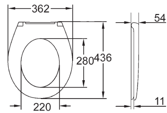
39 492 000 WC-Sitz mit Deckel Quick Release Funktion – werkzeuglos abnehmbar 39 493 000 Soft Close
