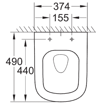
39 206 000 39 206 00H* Wand-Tiefspül-WC kompakt Triple Vortex Spülung randlos
