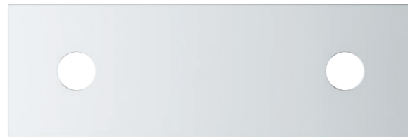
26 785 000 + 26 739 000 | Deckenbrause Abdeckung für 2 Strahlbildner | 334 x 111 mm + Rohbauset | 320 x 100 mm
